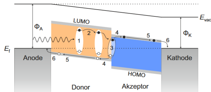
Abb. 14: Das Bild zeigt das Energiediagramm bzw den Ladungstransfer zwischen Donor und Akzeptor-materialeiner organischen Solarzelle. [4]
