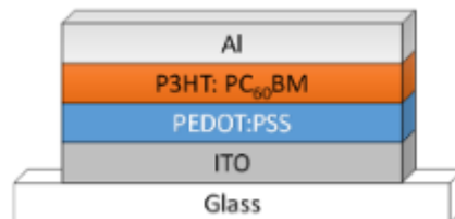
Abb. 13: Das Bild zeigt den strukturellen Aufbau einer organischen P3HT:PCBM basierten Solarzelle. [3]
